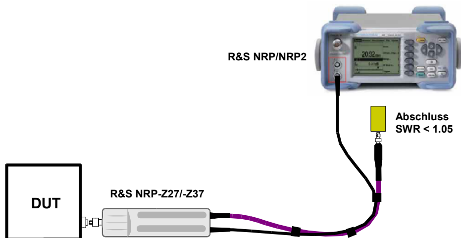
Bild 1-2 Konfiguration mit R&S NRP/NRP2
